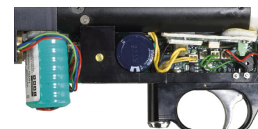
détail de l'unité de contrôle électronique
